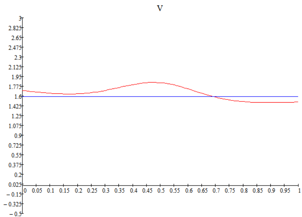
Fig. 6 ( t = 0.5 )
