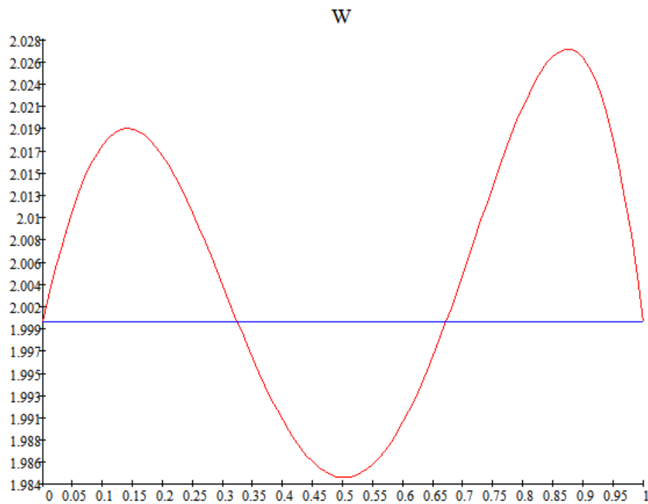
Fig. 13 ( t = 0.138 )
