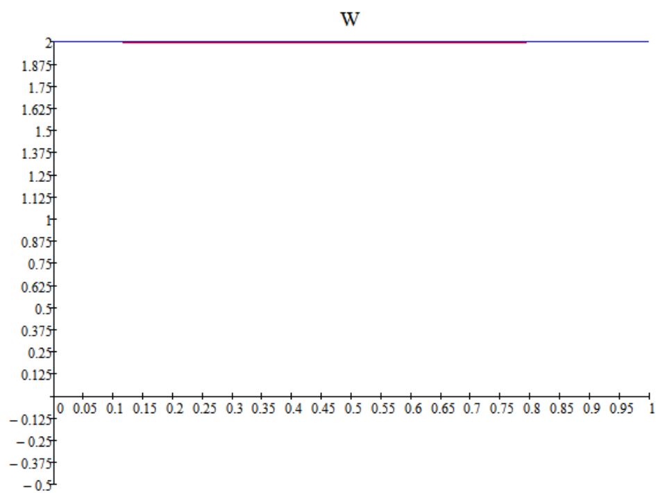
Fig. 7 ( t = 1 )
