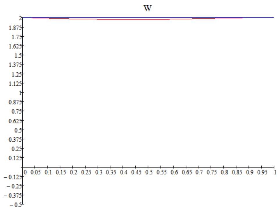
Fig. 5 ( t = 0.5 )
