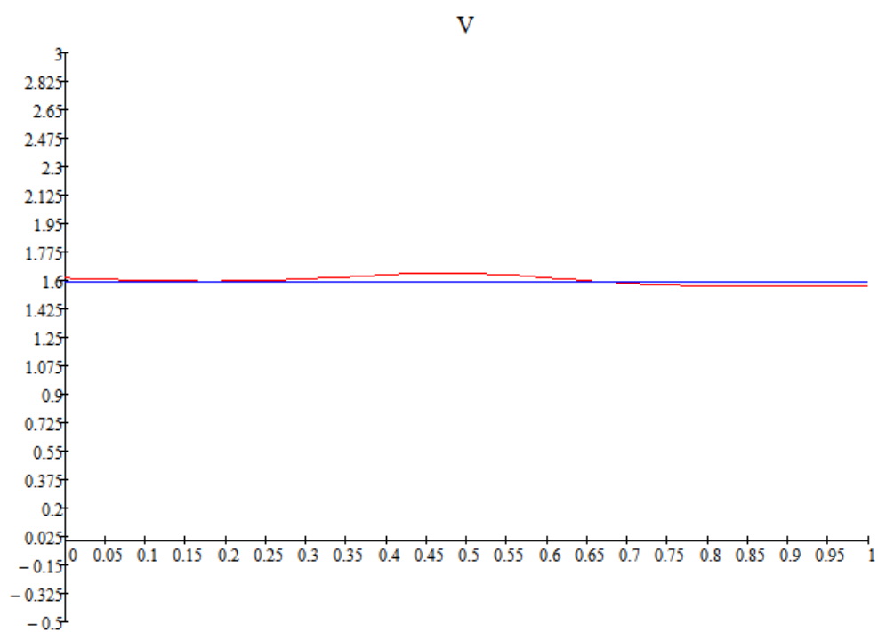
Fig. 8 ( t = 1 )
